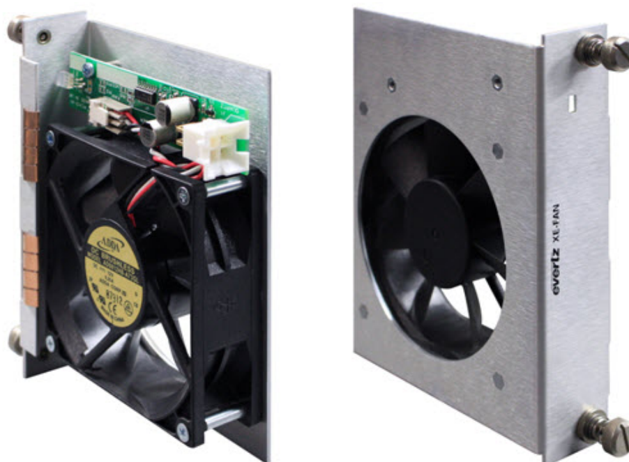
Figure 5-65: Xenon Fan Unit
